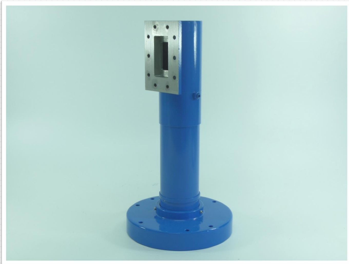
Iluminador Circular Simple Esquerdo 3.625 a 4.200MHz
