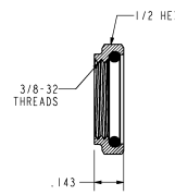
Fig. B Nut Seal
